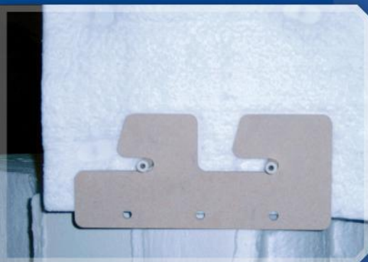
duotherm Modul mit Halterung für Heizungen
